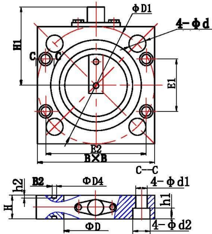
\Phi 100 、 \Phi 125 、 \Phi 150 、 \Phi 200 、 \Phi 250 、 \Phi 300 Plate type valve
