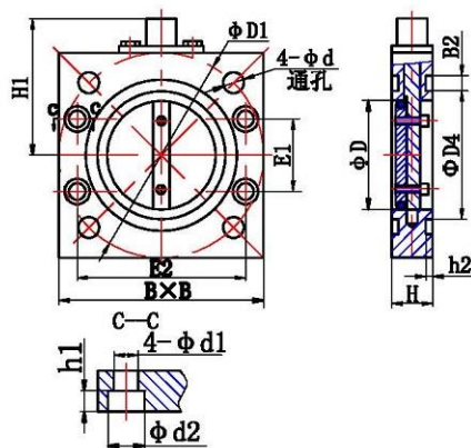
Φ100、Φ125、Φ150、Φ200、Φ250、Φ300 Vacuum valve
