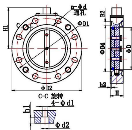
Φ100、Φ125、Φ150、Φ200、Φ250、Φ300 Vacuum valve
